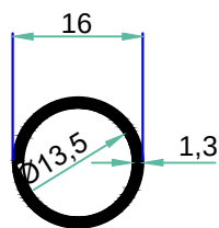
5133 0.157 kg/m
