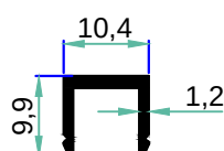
3863 0.035 kg/m
