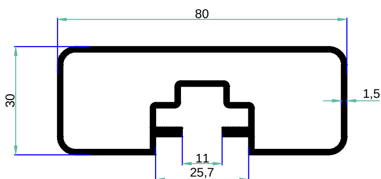
6516 1,089 kg/m
