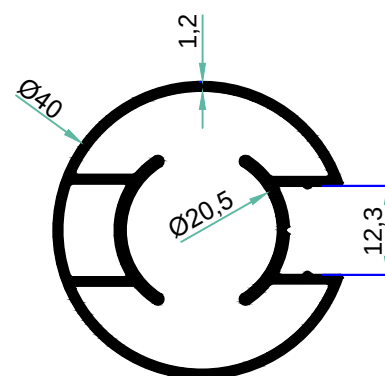
5116 0.650 kg/m
