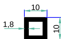
3557 0.160 kg/m
