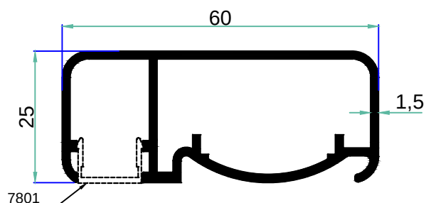
7803 0,776 kg/m
