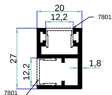
7804 0,393 kg/m
