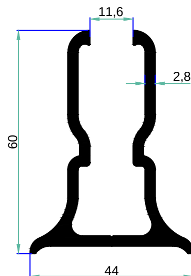
5120 1.303 kg/m
