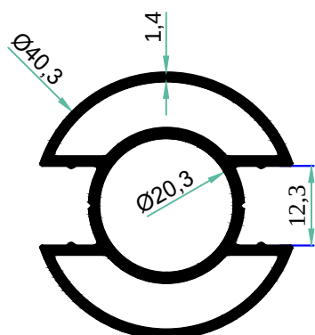
4759 0.795 kg/m
