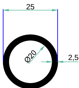
1048 0.478 kg/m
