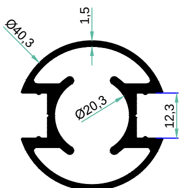
4464 0.890 kg/m
