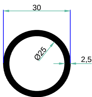
1302 0.585 kg/m
