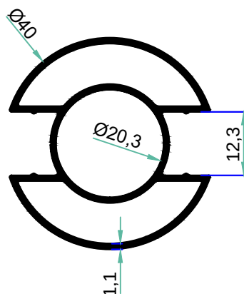
5260 0.593 kg/m
