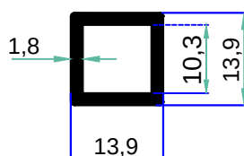
6509 0,235 kg/m
