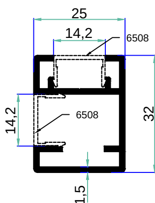
6510 0,472 kg/m
